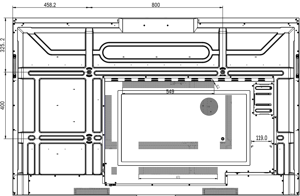
СХЕМА ПАНЕЛИ (ВИД СЗАДИ)
